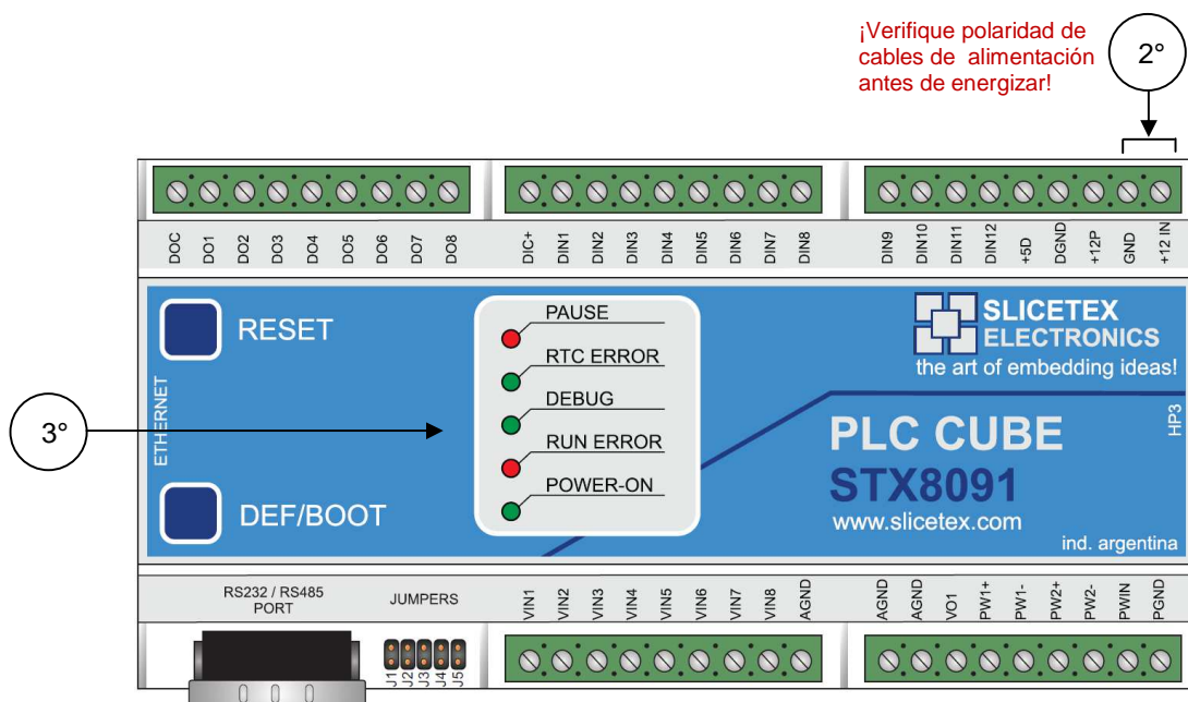
Figura 2: Vista superior mostrando entradas y salidas del dispositivo.
