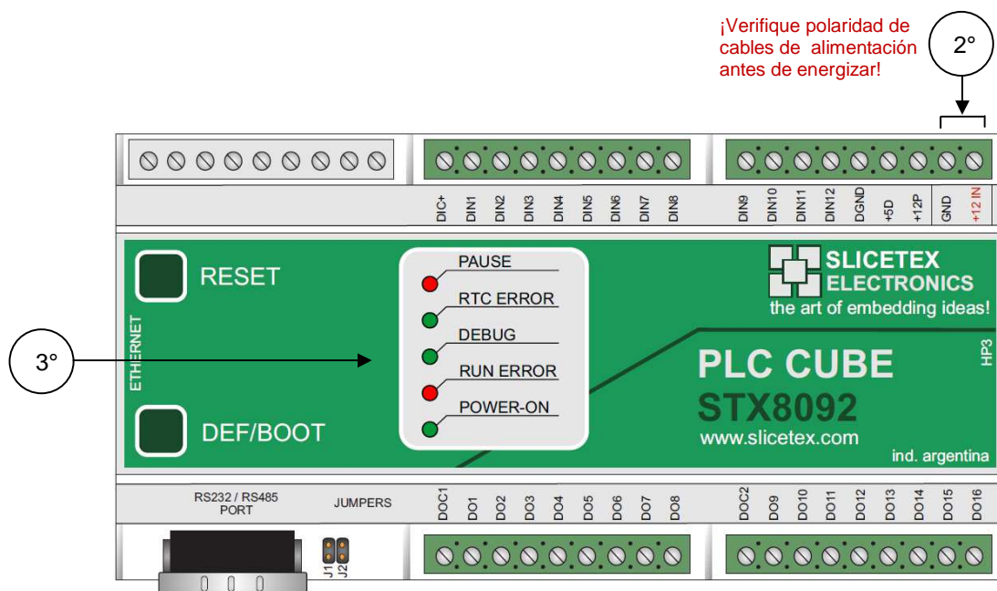
Figura 2: Vista superior mostrando entradas y salidas del dispositivo.
